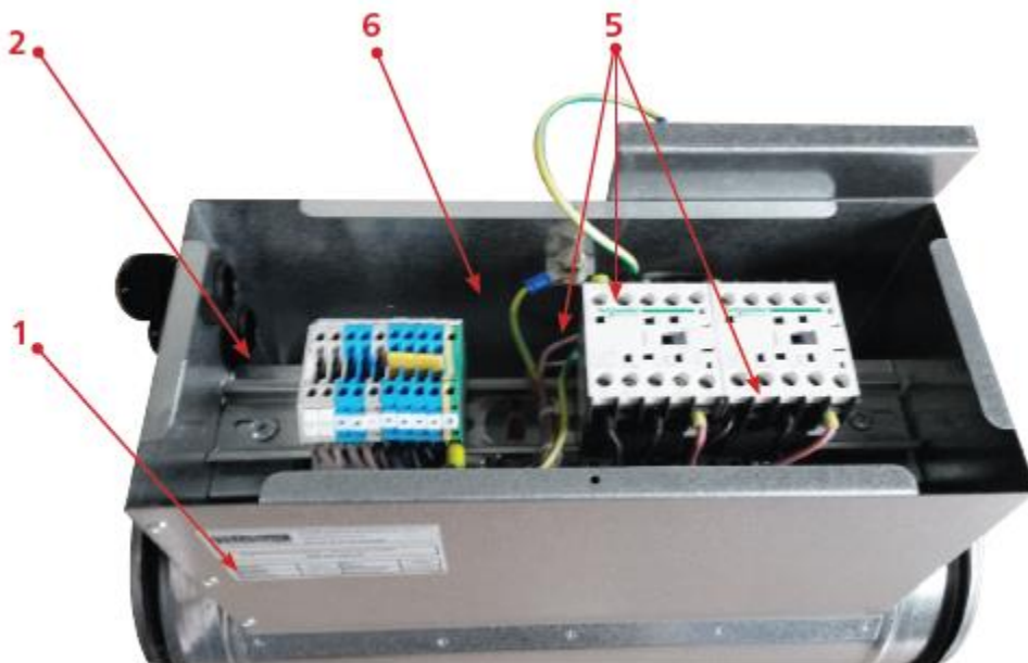
Figure 1 1 Vue générale des radiateurs électriques à gaine circulaire BED-XC
