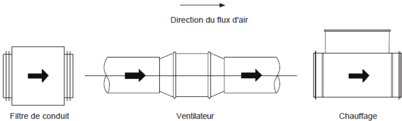
Figure 3 Le schéma de placement des radiateurs électriques à gaine circulaire BED-XC dans une installation.
