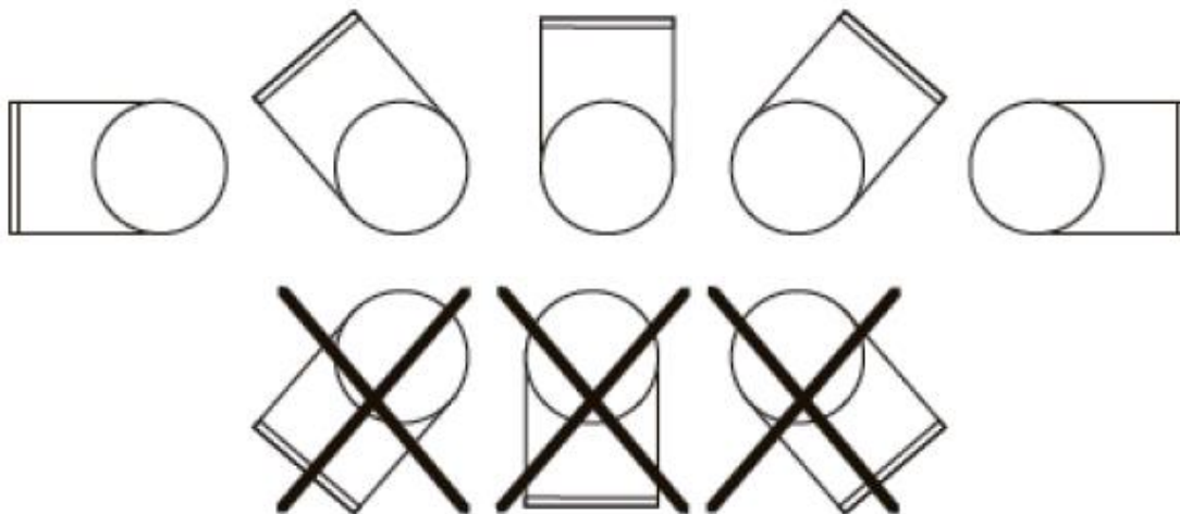
Figure 4 Positions d'installation autorisées des résistances électriques à gaine circulaire BED-XC dans l'installation, par rapport à la position du boîtier de raccordement.
