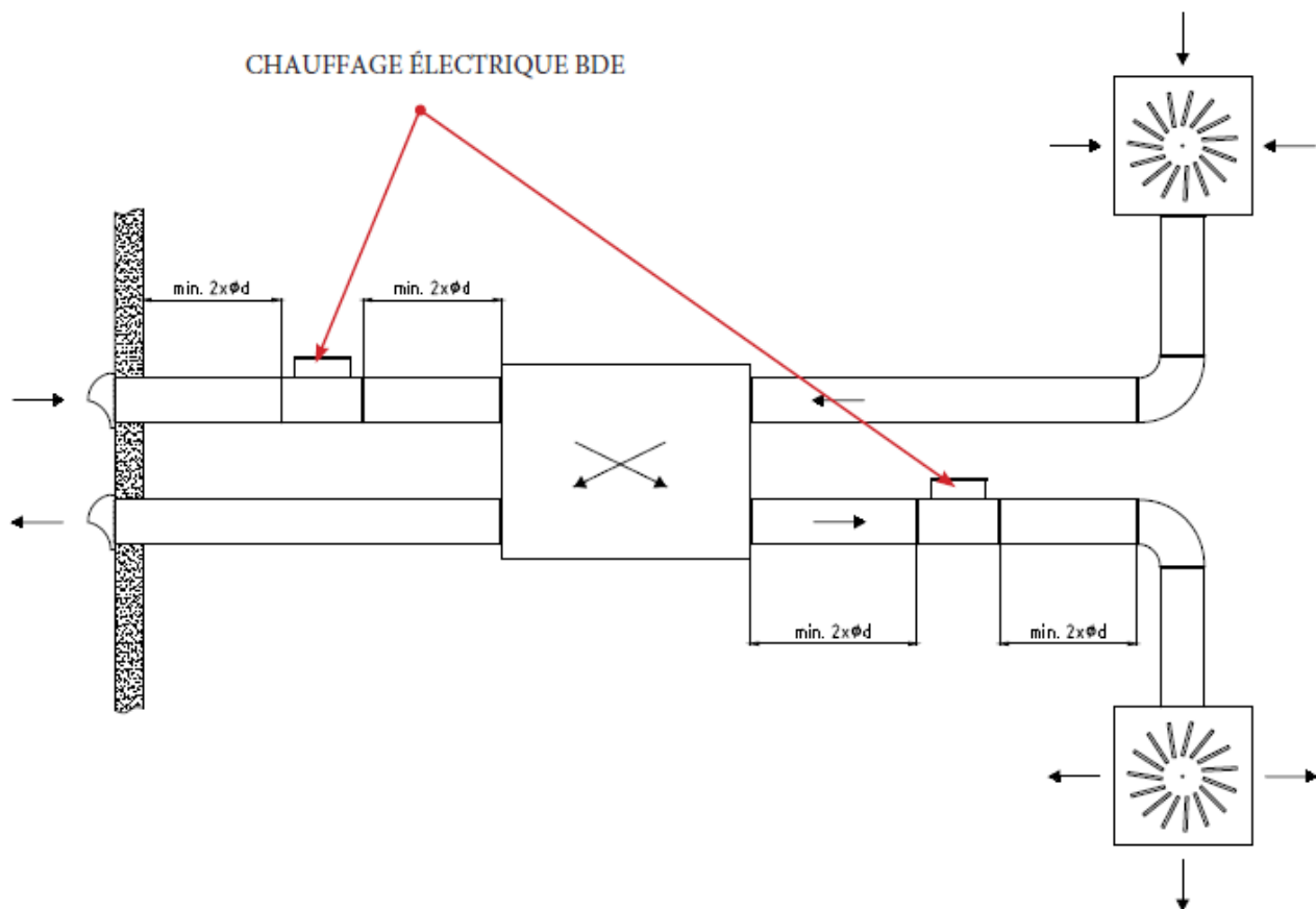
Figure 2 Exemples de lieux d'installation des radiateurs électriques à gaine circulaire BED-XC
