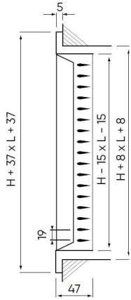
Grille GDD
