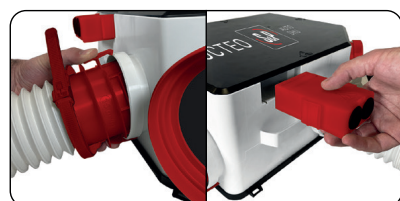
OCTEO® POWERCONNECT Plug&Play - Étanchéité et connectivité jamais égalées
