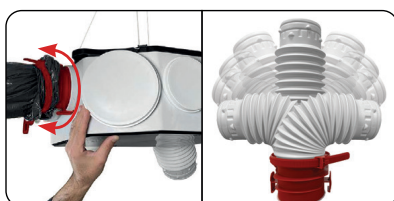
OCTEO® POWERTWIST 360° de possibilités Adaptable et compact
