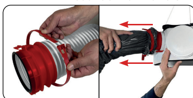
OCTEO® POWERFIX Raccordements simplifiés et ultras résistants
