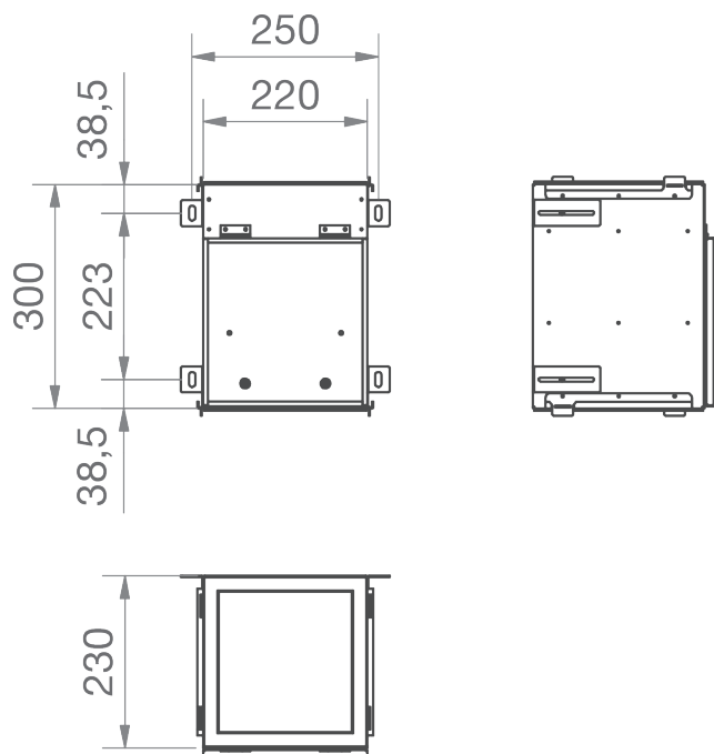
Schémas côtés du caisson filtrant ComfoWell 220
